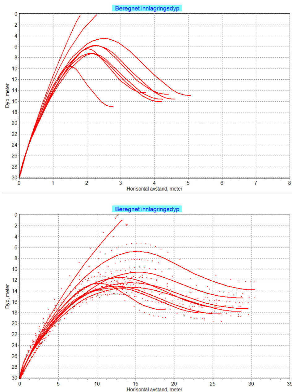
Figur 10. Beregnet innlagringsdyp og fortykning for avløpsvannet fra RA4 ved tidspunktene for prøvetaking. Beregningene er gjort med vannmengden og den vertikale profilen for temperatur og saltholdighet den aktuelle dato. Resultatene påvirkes også av strømhastigheten som varierer med tiden. Øverst er brukt strømhastighet 2 cm/s (en lav hastighet og som er relativt ugunstig mht. innlagring). I nedre figur vises resultatene ved strømhastighet 10 cm/s.
