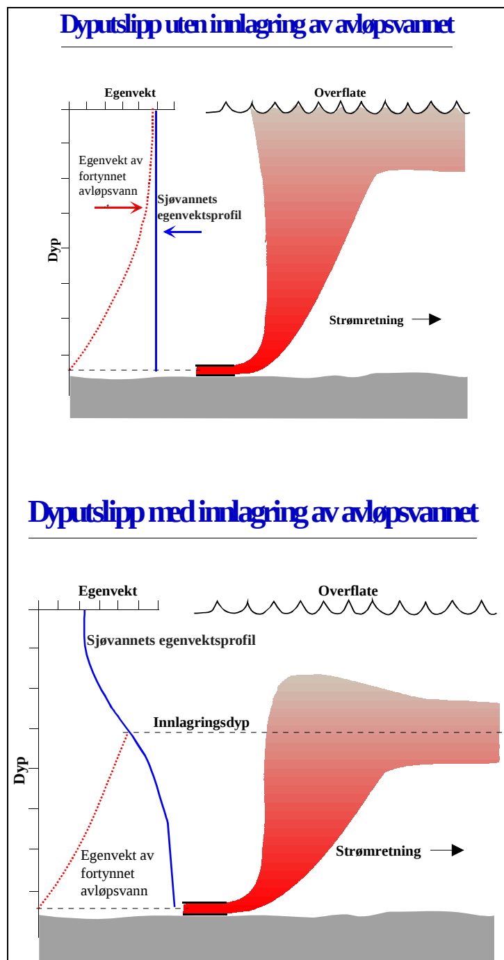
Figur 5. Prinsippskisser som viser hvordan dyputslipp av avløpsvann fungerer i forhold til innlagring. En forutsetning for innlagring er at egenvekten for fjordvannet øker med dypet. Ved den øvre figuren er ikke dette tilfelle og avløpsvannet når til overflata. I den nedre figuren innlagres avløpsvannet.
