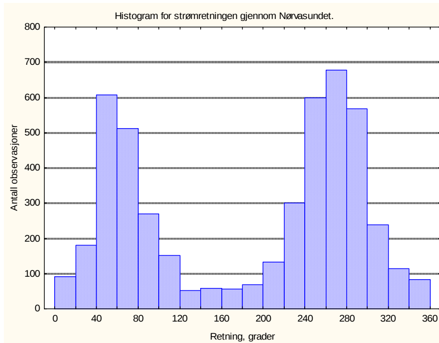
Figur 12. Strømrretningen følger hovedsakelig Nørvasundets lengdeakse, dvs. øst-vest.
