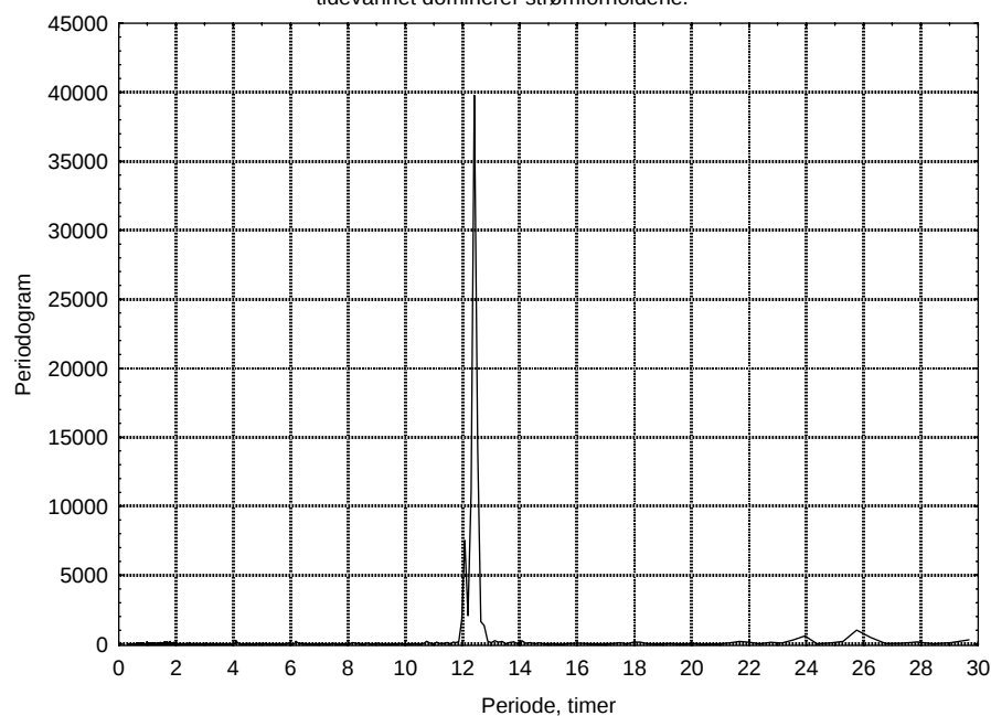
Figur 15. En analyse av variasjoner i strømmens retning og styrke bekrefter at en periode på ca. 12.5 dominerer. Dette viser gjennomstrømningen i stor grad er styrt av det halvdaglige tidevannet.
